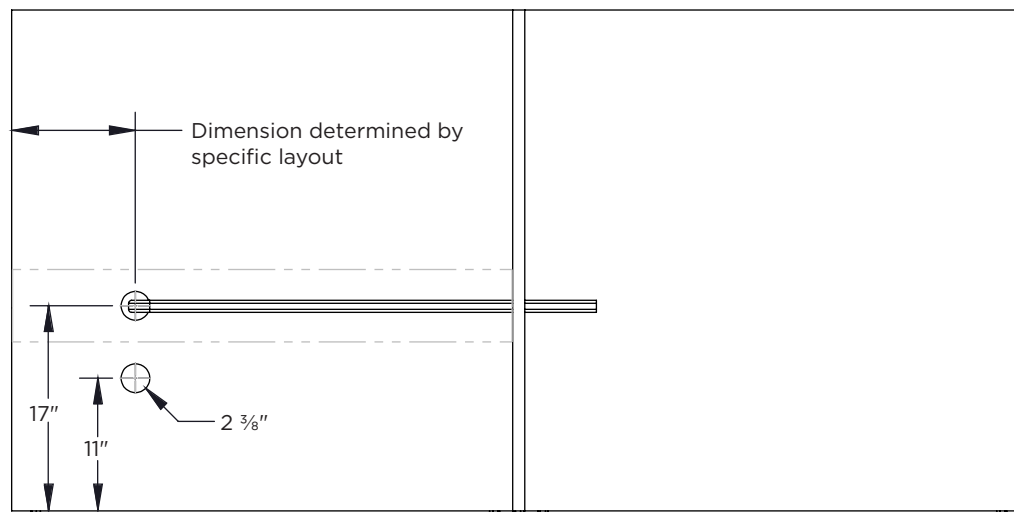
Elevation A
