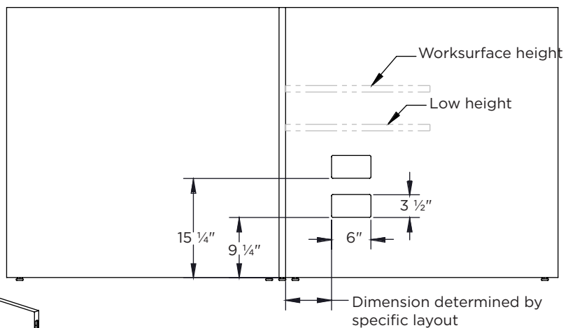
Elevation B
