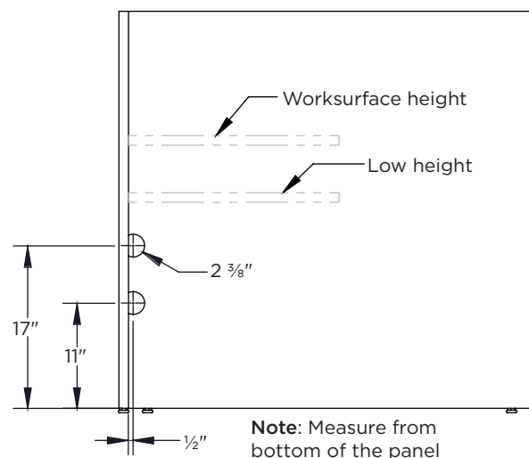
Elevation A
