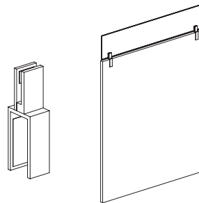
PVPBKT-2 bracket
